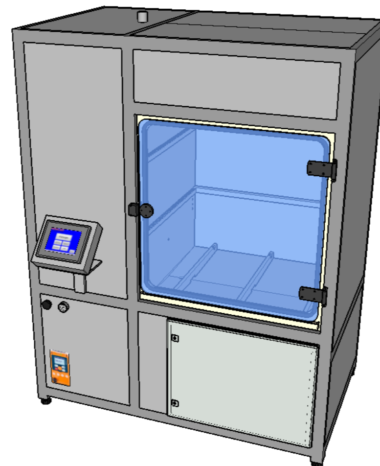
Tür-Ausschnitt 880mmx880mm
